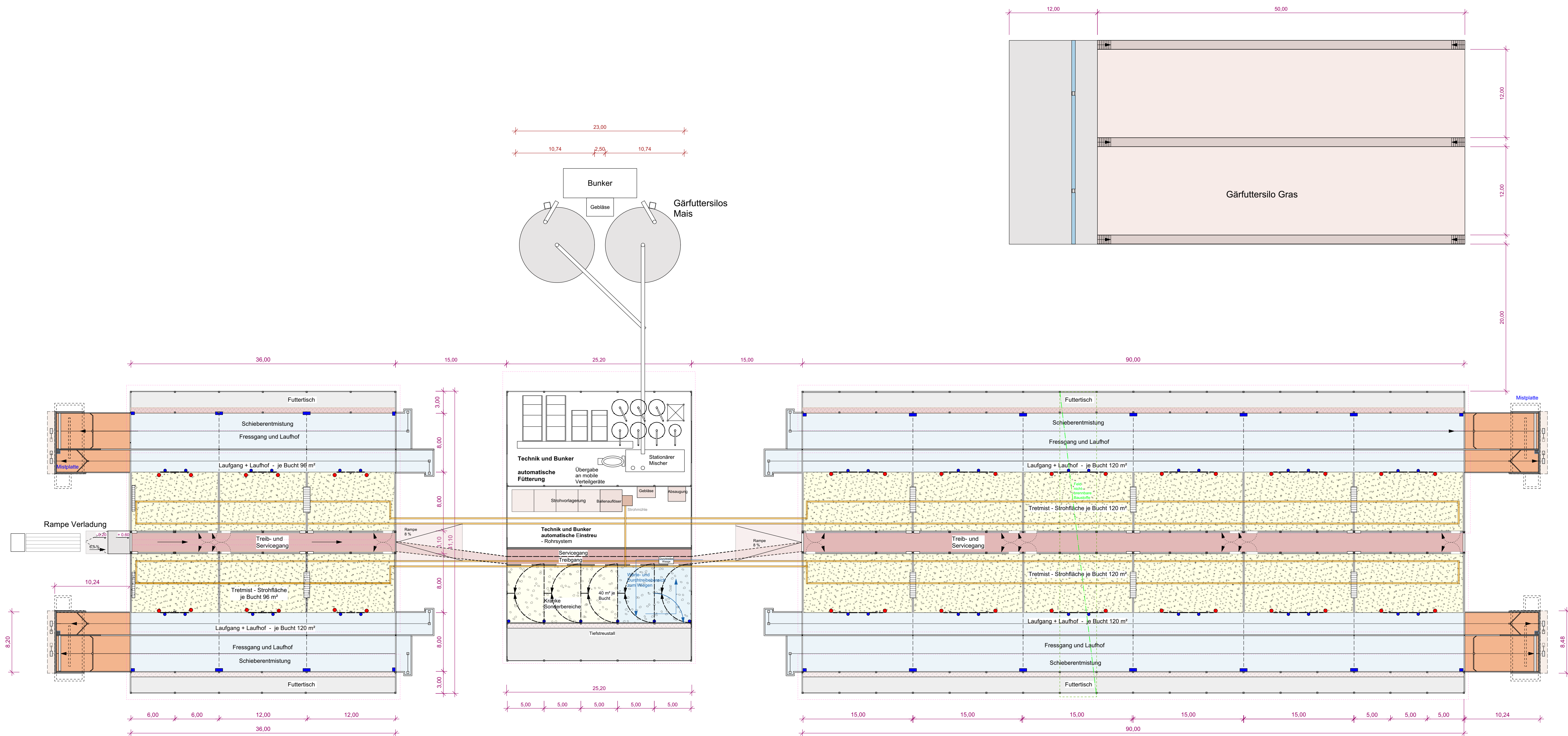
Stallgebäude 2 10 Gruppen > 400 kg
